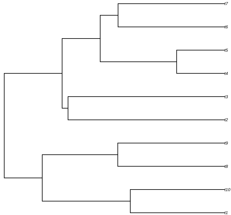
CCD0Beast
