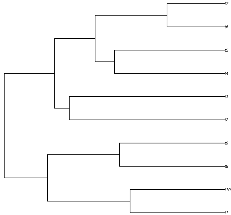
CCD0model
